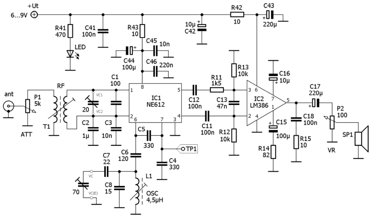
Közvetlen keverésű megfigyelő vevő a 40m-es sávra
